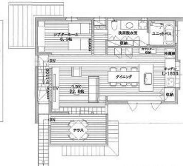
2階平面図 S:1/100
